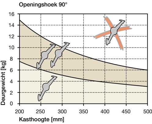
Toepassing Dropdown
